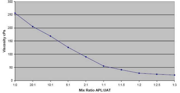
Viscosity Chart APL:UAT
